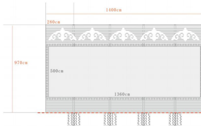
广告牌正面(南)
