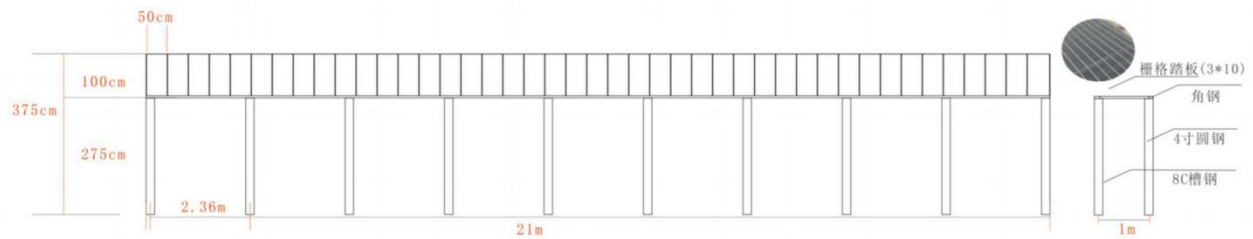
塔顶过道截面图
