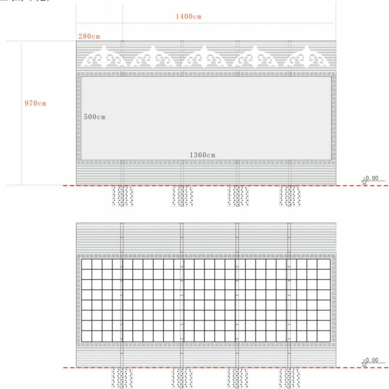
广告牌背面(北)
