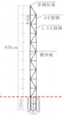
支柱造型侧面结构图(井架)
